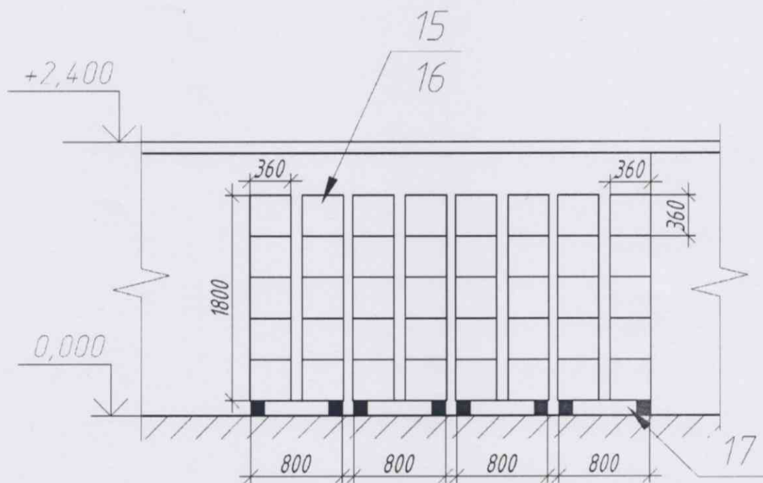
Рис 9 Разрез 6-6
