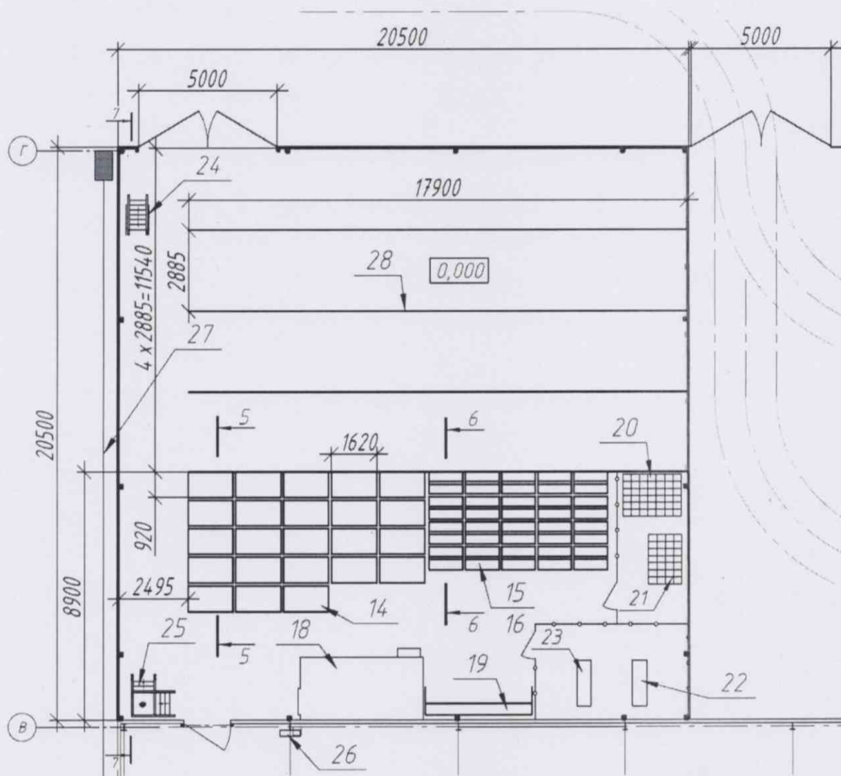
Рис.7 План склада первого этажа
